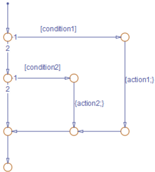
if-elseif
