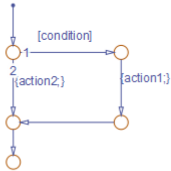
if-else
