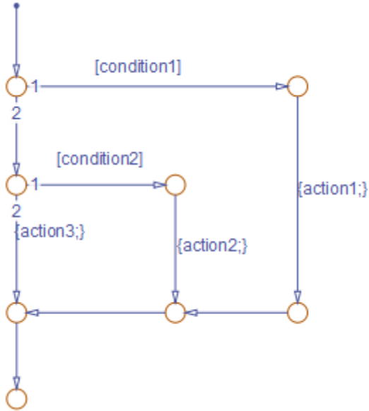
if-elseif-else
